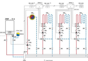
Regulacija vodena spoljnom temperaturom, sa jednim nemešanim krugom i tri kruga grejanja sa mešnim ventilom, tip uređaja ZBR
