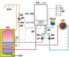
Regulacija vodena spoljnom temperaturom (FW 100) sa jednim krugom grejanja i akumulacionim bojlerom sa recirkulacijom, tip uređaja ZBR
